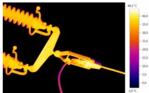
Тепловизионная съемка клеммного соединения изолятора (расстояние до объекта примерно 15 м)
